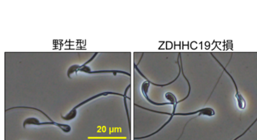
図 3. マウス精子の形態
