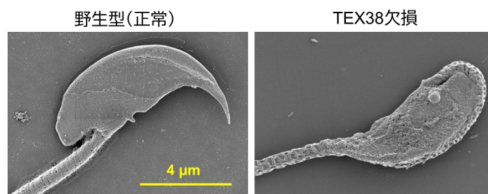
図1. マウス精子頭部の電子顕微鏡像
