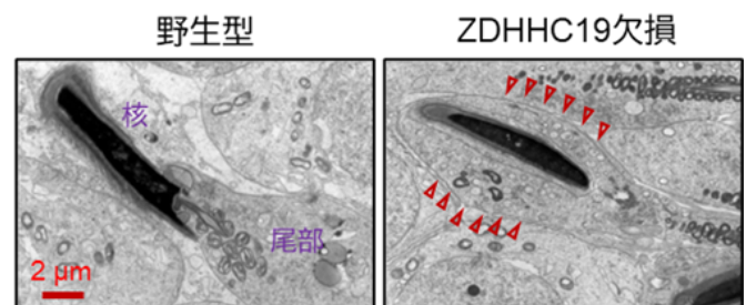
図 4. 精巣内の精子完成直前の電子顕微鏡観察像
