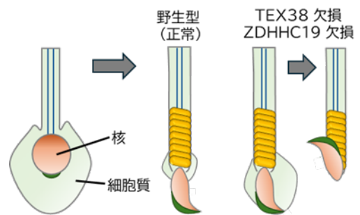
図 5. 精子形成における細胞質の除去
