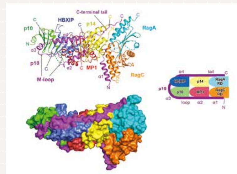
図2：mTORを制御するRagulator複合体タンパク質群の結晶構造
