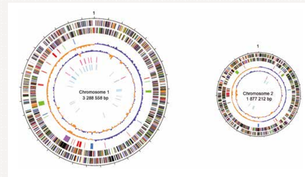
図1：腸炎ビブリオのゲノム解析。 腸炎ビブリオを始めとするビブリオ属細菌のゲノムは、2つの環状染色体より構成される。
